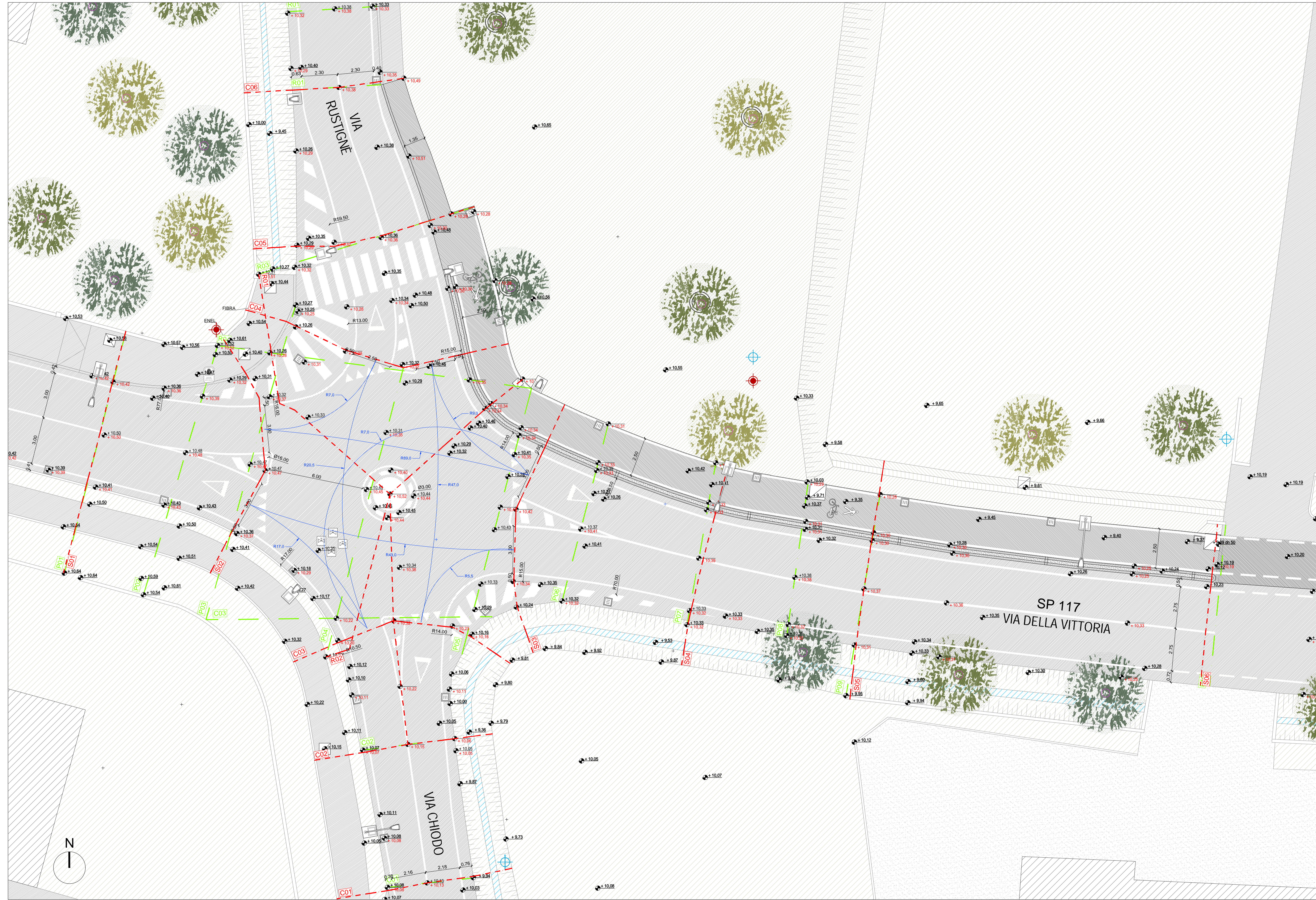
Planimetria generale - Stato di Progetto - scala: 1:100
